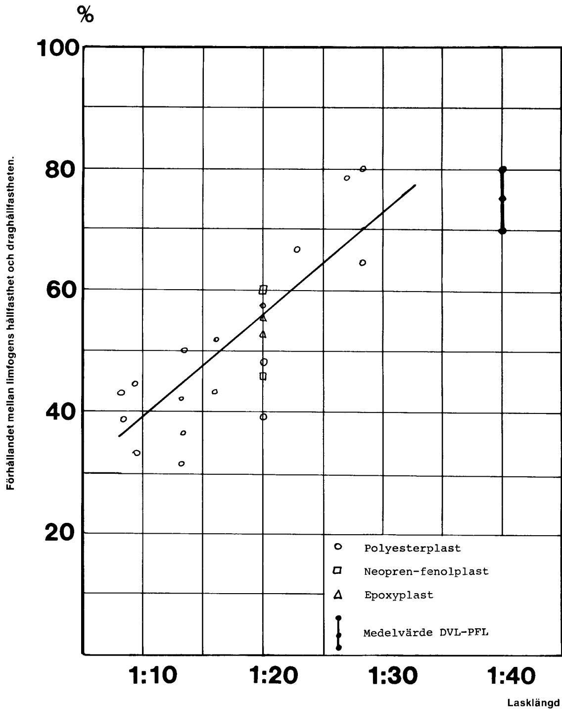
Limhållfasthet vid dragbelastning och laskade laminatprov Glasfiberväv 112 och 181
